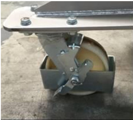
Roues arriere pivotantes nylon Frein papillon
