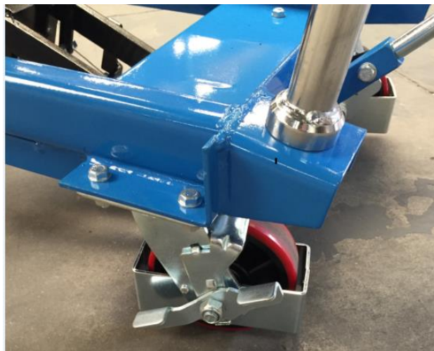
Detail roue pivotante avec frein papillon et fixation poignée
